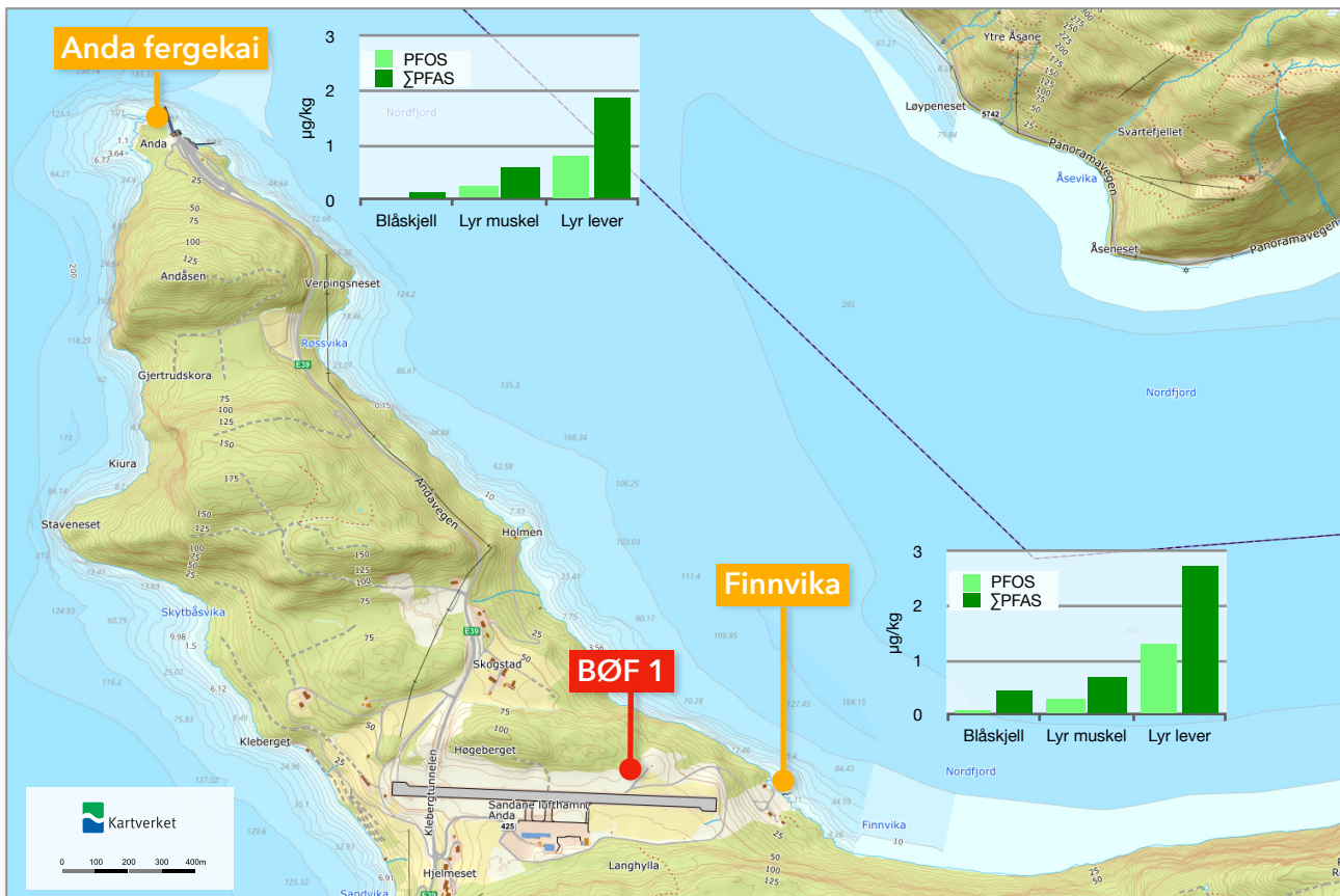
Figur 5. Kart som viser de enkelte stasjonene for innsamling av lyr og blåskjell ved Sandane lufthavn i august 2023. Brannøvingsfeltet BØF 1, som drenerer mot Finnvika, er markert med rød sirkel. Søylediagrammene viser midlere konsentrasjoner av PFOS og sum av 26 PFAS-forbindelser ( \Sigma PFAS) i de ulike prøvetypene
