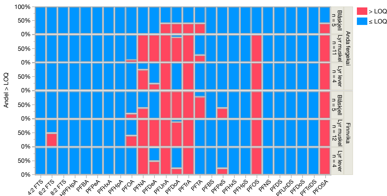
Figur 3. Andelen av biotaprøver med kvantifiserbare konsentrasjoner (>LOQ) av de ulike PFAS-forbindelsene fra stasjonen Finnvika ved Sandane lufthavn og referansestasjonen ved Anda fergekai. Materialet ble innsamlet i august 2023.
