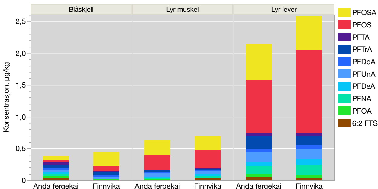
Figur 4. Midlere konsentrasjoner av utvalgte PFAS-forbindelser i biotaprøver fra stasjonen Finnika ved Sandane lufthavn og referansestasjonen ved Anda fergekai. Konsentrasjoner under kvantifikasjonsgrensen ( \leq LOQ) er erstattet med halve grensen (LOQ/2). Materialet ble innsamlet i august 2023.
