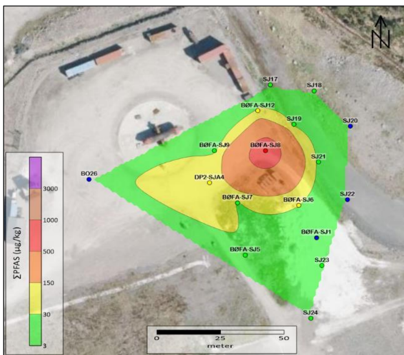
Figur 27 Interpolert konsentrasjonsfordeling av \Sigma PFAS generert av programvaren Surfer basert på \Sigma PFAS-konsentrasjoner i 2-3 m dybde per prøvepunkt. Figuren inkluderer prøvetakingspunkter fra DP2-undersøkelsen i 2011, samt supplerende undersøkelser i 2020-2021.
