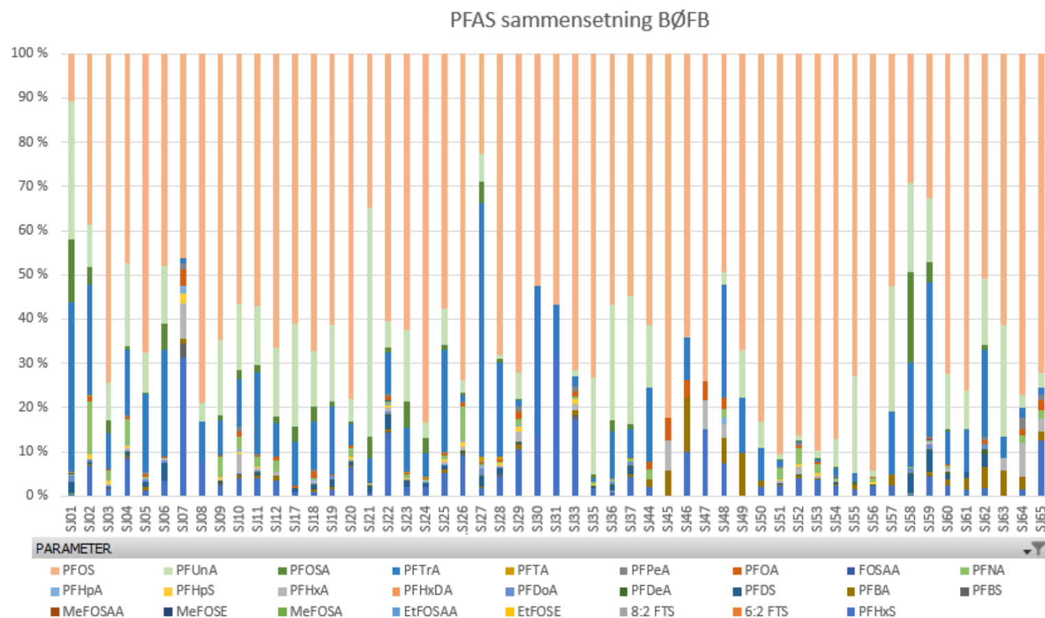
Figur 44 PFAS-sammensetning i jordprøver fra BØFB, prøvetatt i 2021-2022. Det er kun parametere som er påvist i minst én av prøvene som er vist i figuren. Resultater er vist som gjennomsnittlig prosentvis konsentrasjonsfordeling av de ulike PFAS-forbindelsene per prøve.
