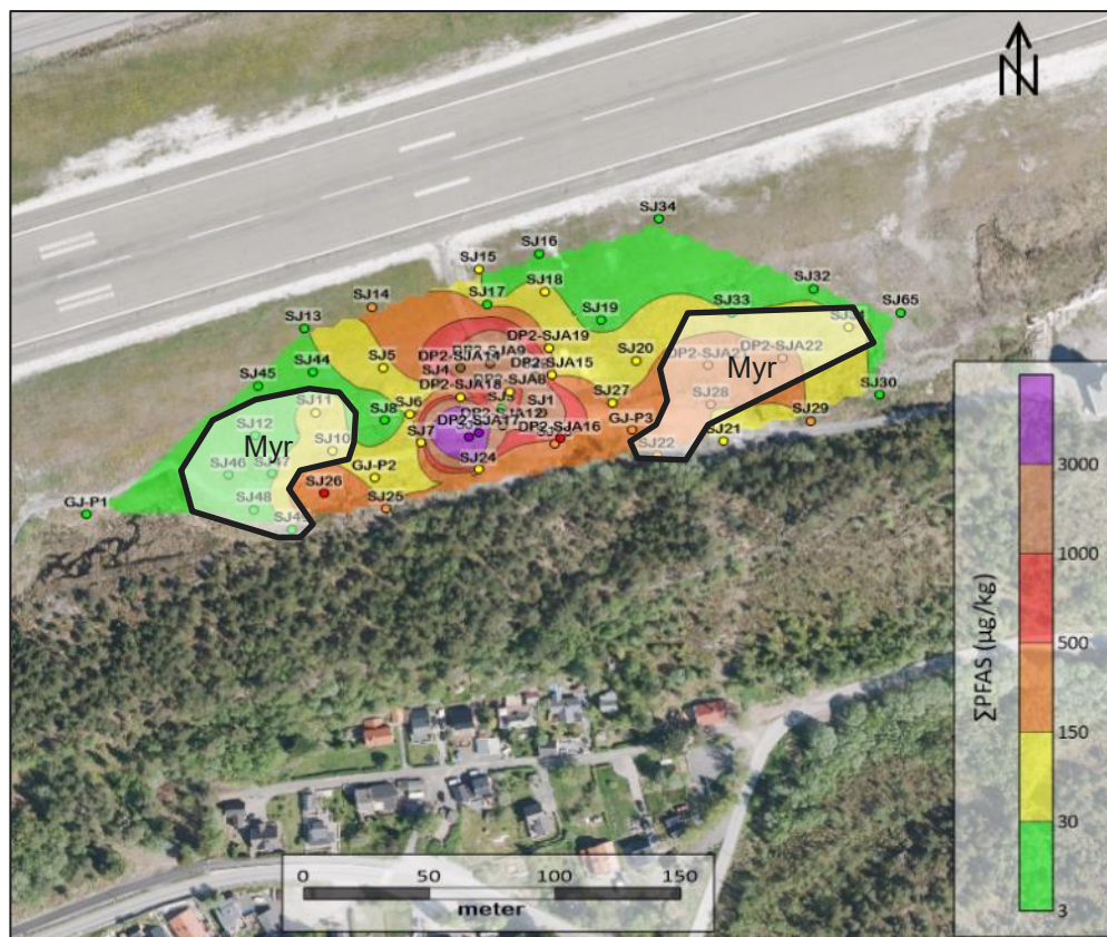
Figur 73 Interpolert konsentrasjonsfordeling av \Sigma PFAS ( \mu\text{g/kg} ) i overflatejord (0-1 m) på BØFB flaten, basert på analyseresultater fra 2011-2022. Med utgangspunkt i feltobservasjoner (Figur 32), er antatt utstrekning av myrjordmasser vist.
