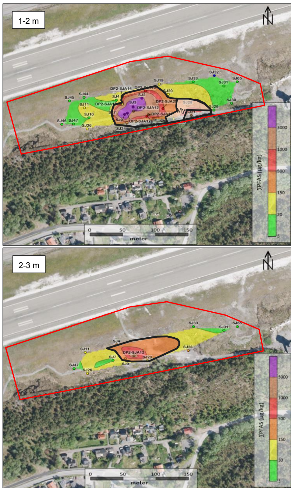
Figur 76 Interpolert konsentrasjonsfordeling av \Sigma PFAS ( \mu\text{g/kg} ) for 1-2 m (øverst) og 2-3 m (nederst) dybde på BØFB flaten, basert på analyseresultater fra 2011-2022. Foreslått graveområde med tiltaksgrense >150 \mu\text{g/kg} er vist med sort linje, og antatt utstrekning av myrjordmasser innenfor foreslått tiltaksgrense er vist. Omtrentlig plassering av tiltaksområdet er vist med rødt omriss.
