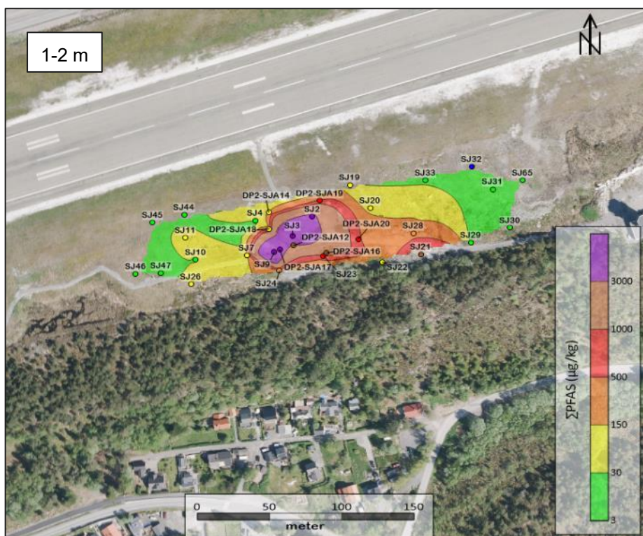
Figur 40 Interpolert konsentrasjonsfordeling av \Sigma PFAS i jord ( \mu\text{g/kg} ) på BØFB flaten, basert på analyseresultater fra 2011-2022. Figuren er basert på prøver fra 1-2 m dyp.
