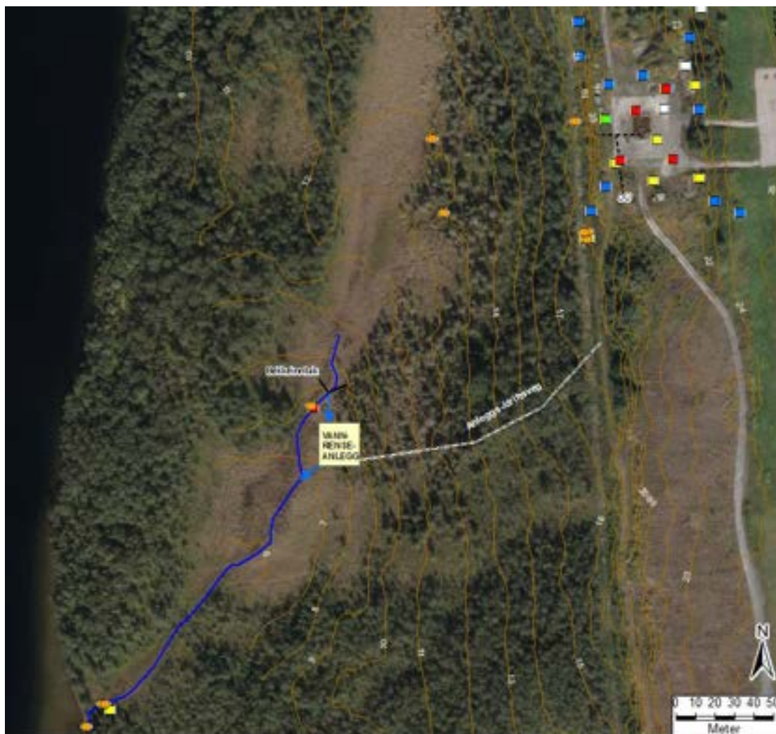
Figur 4-4: Skissert løsning for rensing av bekkevann. Det etableres anleggs-/driftsveg fra eksisterende driftsveg på lufthavnen.
