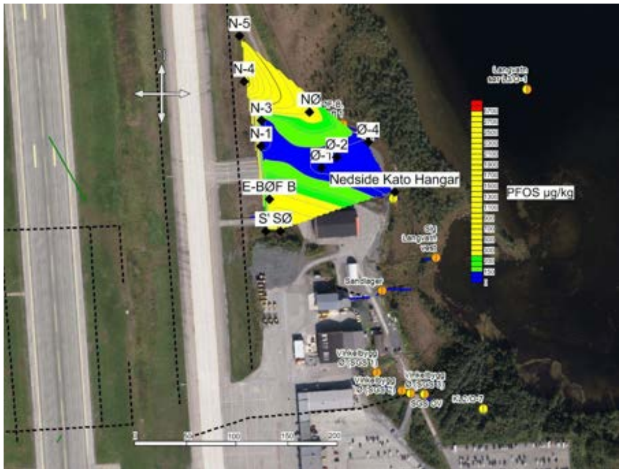
Figur 2-3: Viser interpolert PFOS-konsentrasjon i jord på og rundt BØF B for alle prøvene som er analysert. Interpoleringen er gjort i programvaren Surfer og interpoleringsmetoden som er brukt er "natural neighbour". Overvannssystem er markert med sort stiplede linje.
