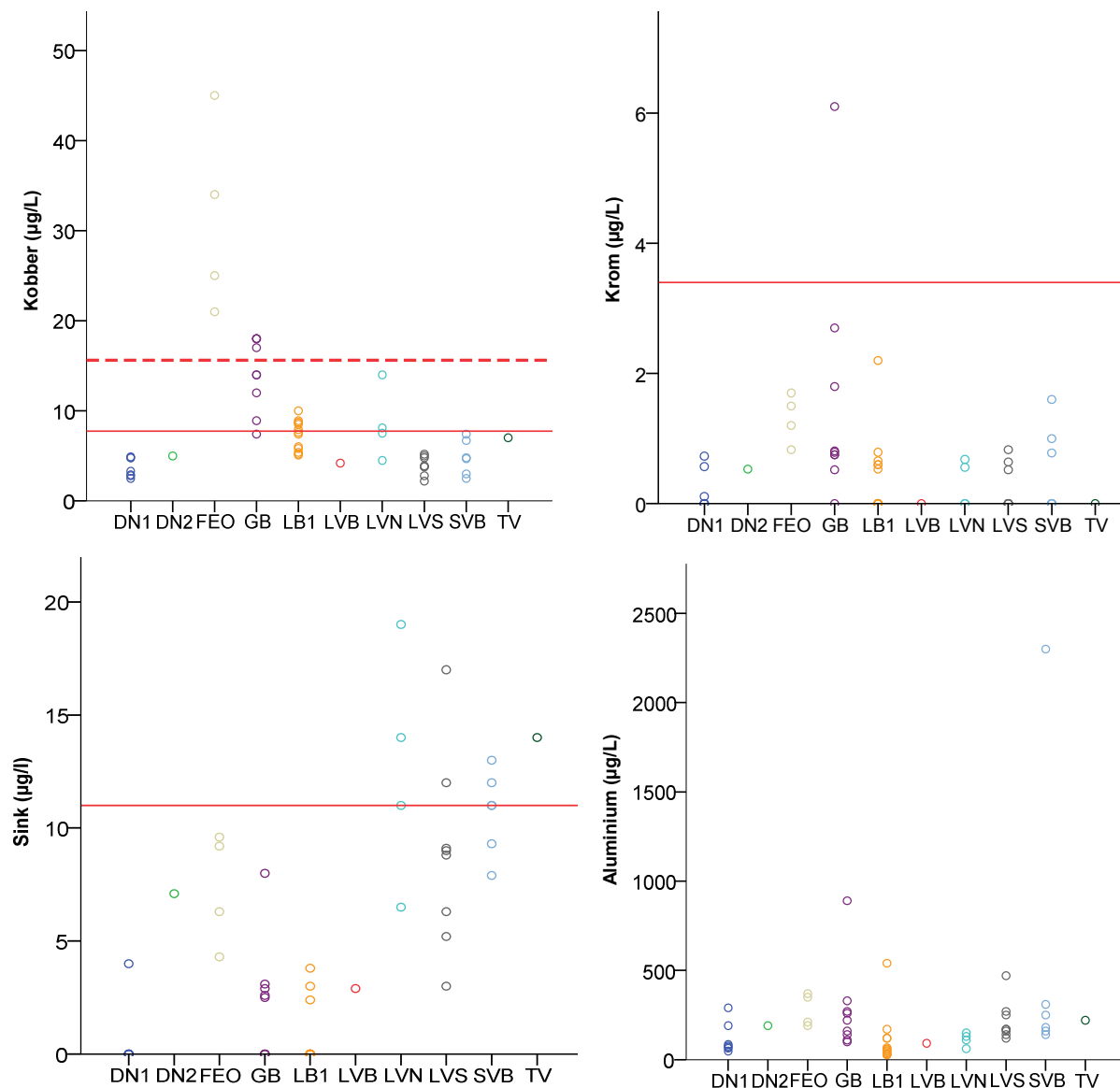
Figur 3.5. Konsentrasjoner (µg/L) av kobber, krom, sink og aluminium i elver og tjern fra Bergen Lufthavn Flesland, og referanseområdet Træsvatn. Rød, heltrukken linje markerer grenseverdien for akutt og kronisk toksisitet (AA-EQS og MAC-EQS er sammenfallende for kobber, krom og sink). For aluminium er det ikke oppgitt grenseverdier, da toksisiteten er avhengig av pH. Rød stiplet linje markerer grenseverdien mellom tilstandsklasse IV -Dårlig, og V- Svært dårlig. Over linjen er det i henhold til veiledere fare for omfattende akutt toksisitet for vannlevende organismer. DN= Deponi Nord, FEO=Fleslandselven Øvre, GB= Gåstjørnsbekken, LB1= Lønningsbekken, LVB= Lindevikabekken, LVN= Langavatn Nord, LVS=Langavatn Sør, SVB=Storaveitabekken, TV= Træsvatn.
