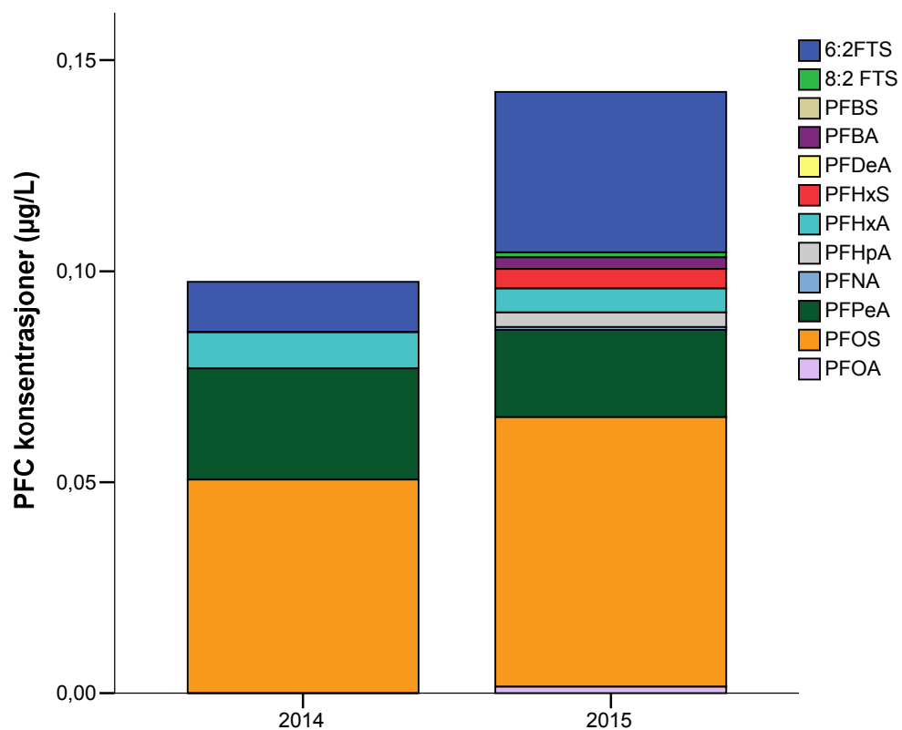
Figur 3.2. Gjennomsnittkonsentrasjoner (µg/L) av perfluorerte forbindelser i vann for 2014 og 2015 ved stasjon Langavatn Øst som ligger nærmest det nåværende brannøvingfeltet ved Bergen Lufthavn Flesland.
