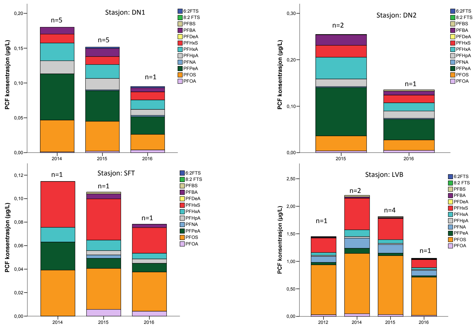
Figur 3.3. Gjennomsnittskonsentrasjoner per år for perfluorerte forbindelser i vann (µg/L) ved utvalgte stasjoner ved Bergen Lufthavn Flesland i perioden 2014-2016. n= antall målinger som snittet er basert på. Stasjonsnavn: DN =Deponi Nord, SFT = Steinfjelltjern, LVB = Lindevikabekken.
